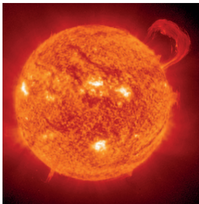
Een grote uitbarsting op de Zon, vastgelegd door de Europese/Amerikaanse ruimtetelescoop SOHO (Solar and Heliospheric Observatory)
