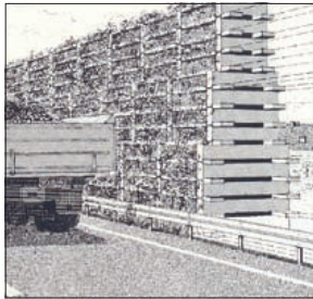
De 'groene' wand van Ebensee bestaat uit een betonnen constructie. Deze wordt met behulp van losse elementen trapsgewijs opgebouwd. Hierdoor is het mogelijk om met een basisbreedte van 1.80 m een hoogte van 9 meter te bereiken. De ontstane ruimten in de 'open' trap worden opgevuld met aarde waardoor een begroenbare wand verkregen wordt. Om de aarde vochtig te houden is op twee hoogtes een bevoeiingssysteem ingebouwd.
