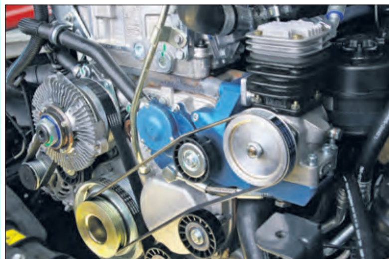
Bij het hier getoonde motorblok is duidelijk met de kleuren blauw, zilver en goud de luchtcompressor te zien die er door de firma Veldhuizen is ingebouwd om zo de bestelauto van luchtremmen te voorzien.
